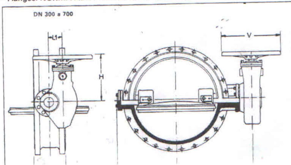
VALVULA BORBOLETA C/ FLANGE REDUTOR E VOLANTE.
